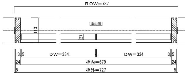
■横断面図
