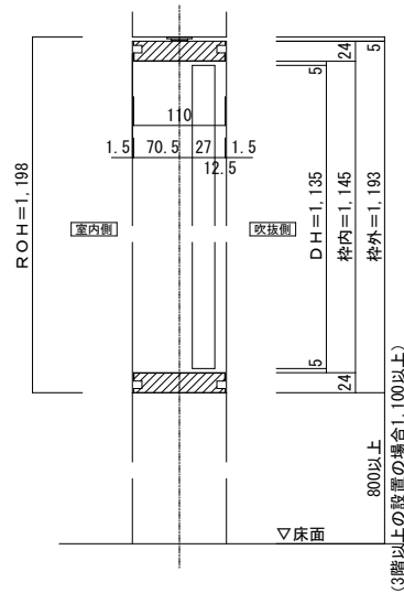
■縦断面図
