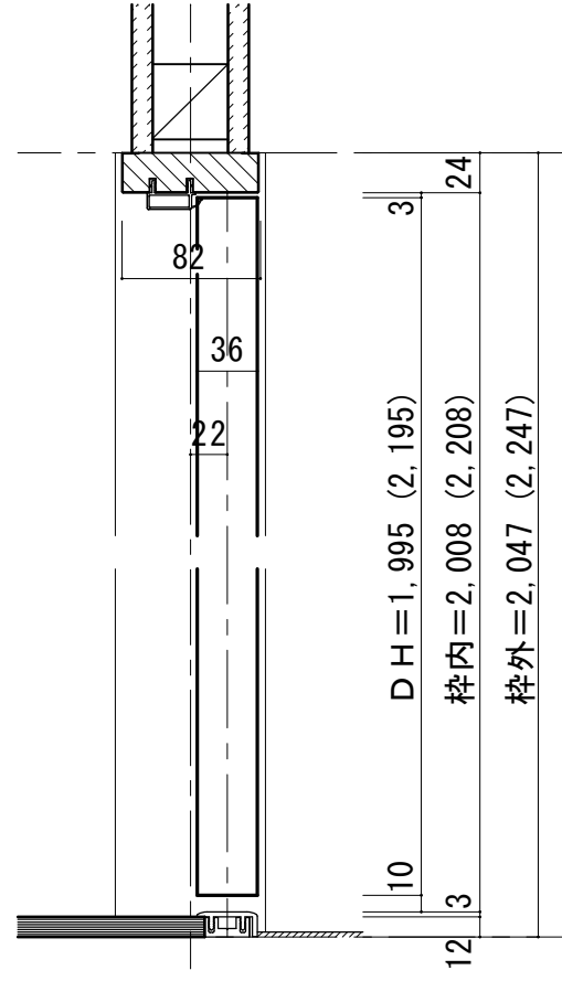
■縦断面図 [片ツパタイプ]
