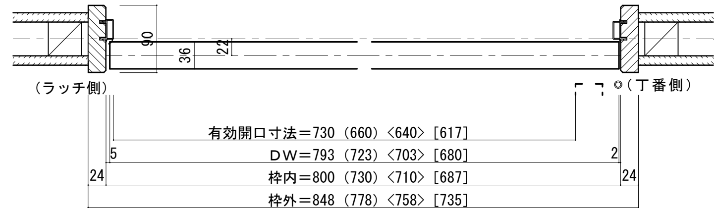
■横断面図
