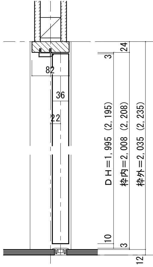
■縦断面図 [両ツパタイプ]
