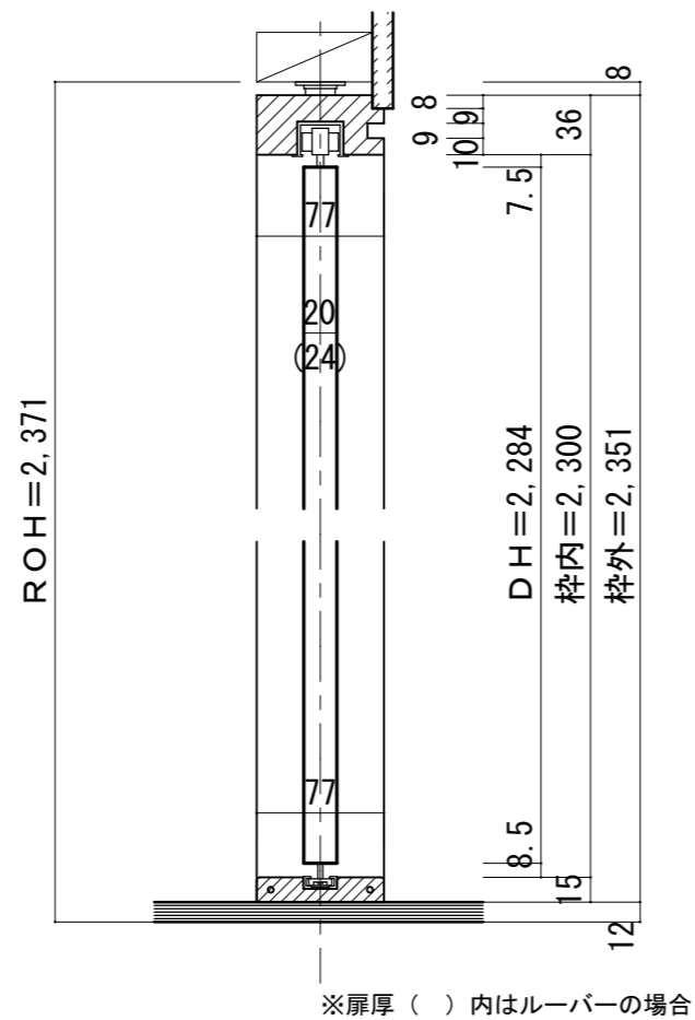
■縦断面図
