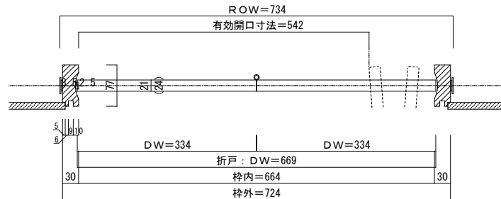
■横断面図
