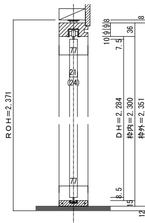
■縦断面図
