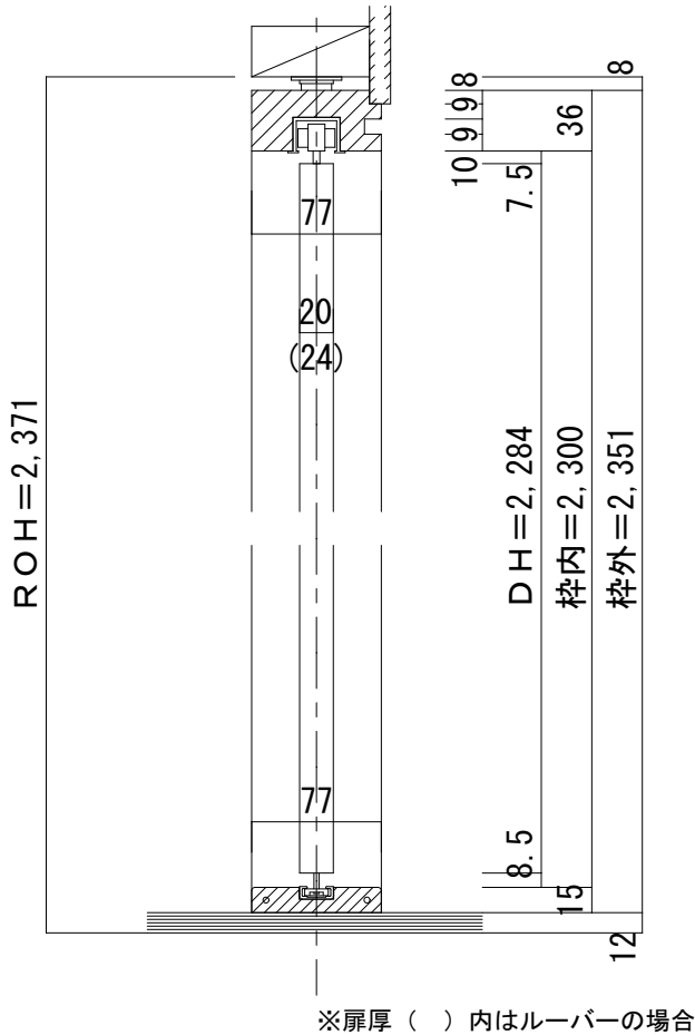
■縦断面図
