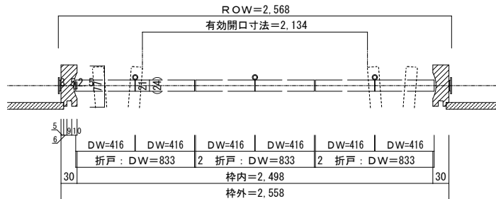
■ 横断面図
