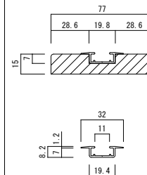
下枠詳細図 (S=1/2)
