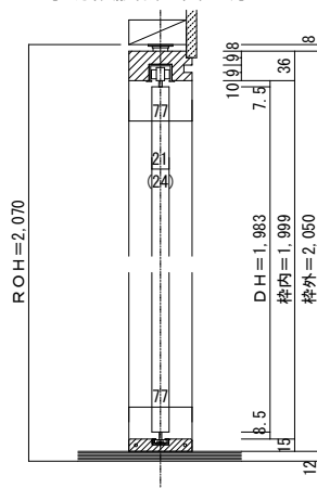
■縦断面図
