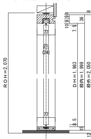
■縦断面図
