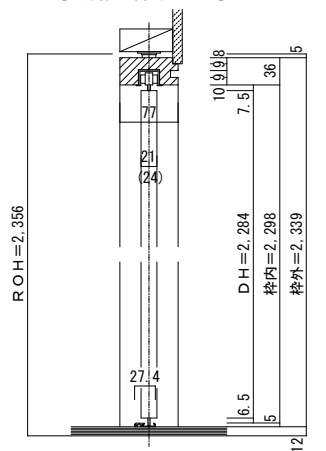
■縦断面図
