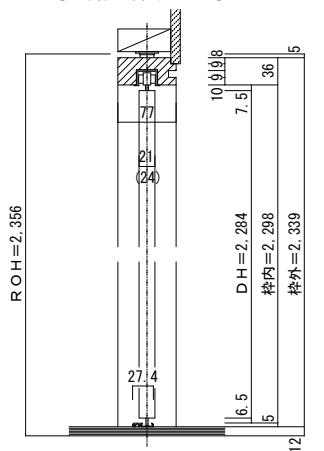
■縦断面図
