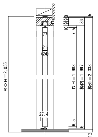
■縦断面図 [3方枠+床直付レール]
