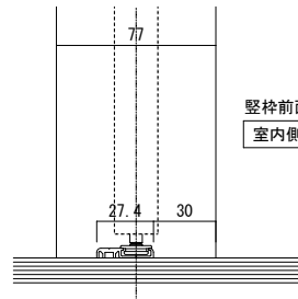
床直付レール取り付け位置 (S=1/2)
