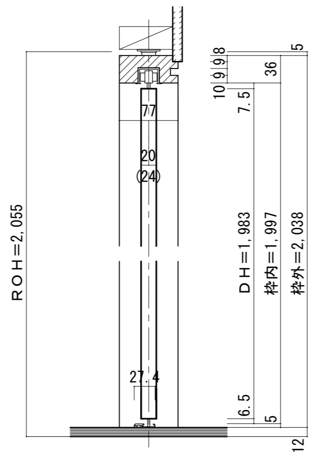
■縦断面図 [3方枠+床直付レール]
