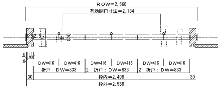
■横断面図
