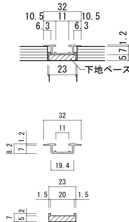
■ レール拡大図 (S=1/2)
