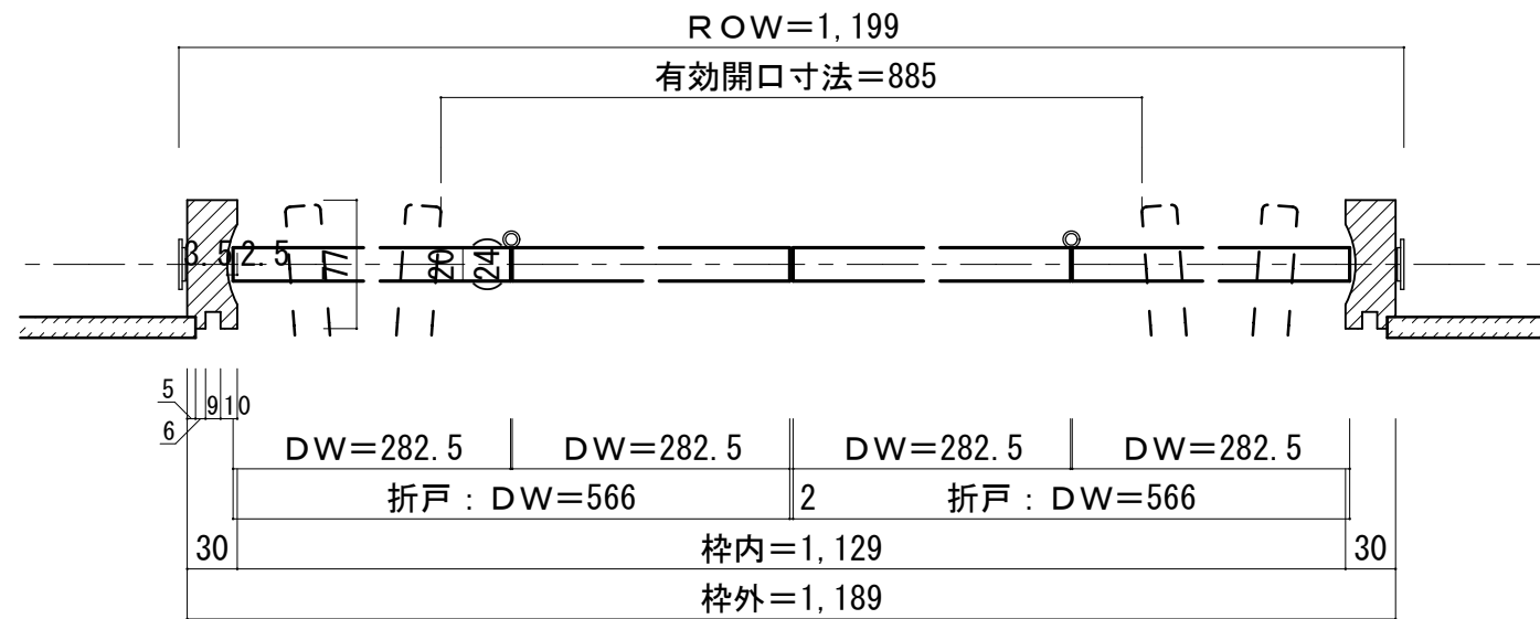
■横断面図
