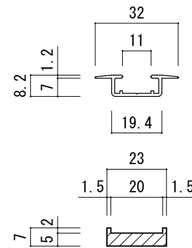
レール埋込時 フロアー貼込位置
