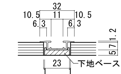
レール拡大図 (S=1/2)
