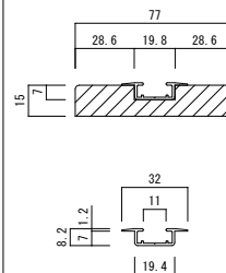
下枠詳細図 (S=1/2)
