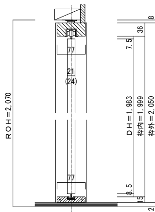
■縦断面図
