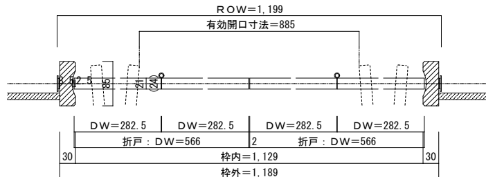
■横断面図
