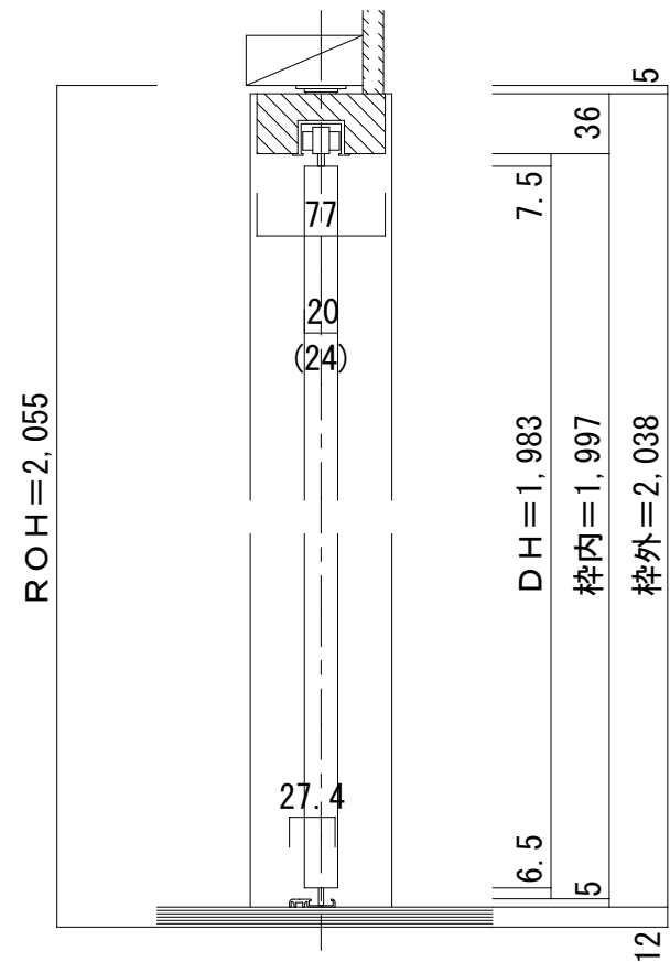
■縦断面図
