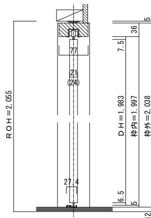
■縦断面図
