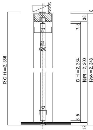
■縦断面図
