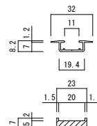
レール埋込時 フロアー貼込位置
