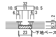
レール拡大図 (S=1/2)
