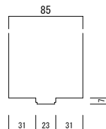
竖枠下端形状図 (S=1/3)
