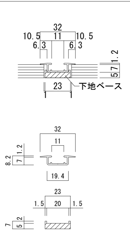
■ レール拡大図 (S=1/2)
