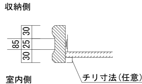
レール埋込時 フロアー貼込位置
