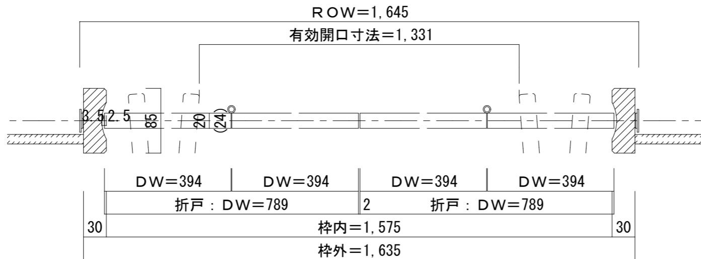
■横断面図
