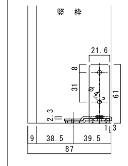
土間金具取付位置 S=1/2
