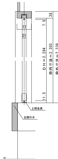
■縦断面図
