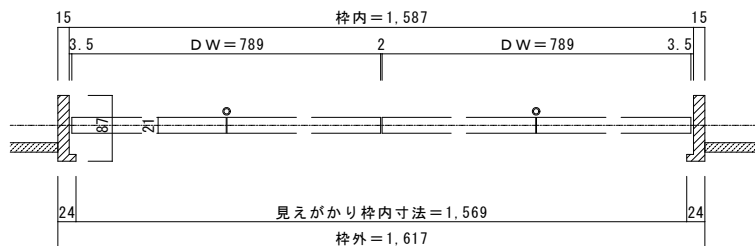
■横断面図[間口6尺]
