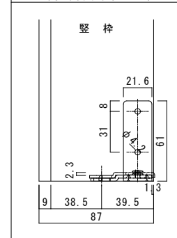
土間金具取付位置 S=1/2
