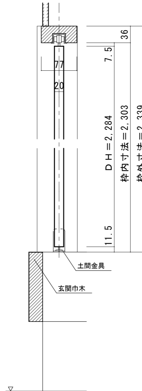
■縦断面図
