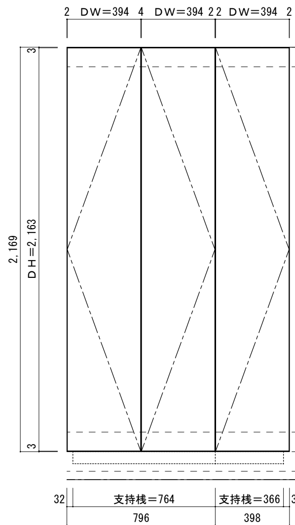
扉配置図
