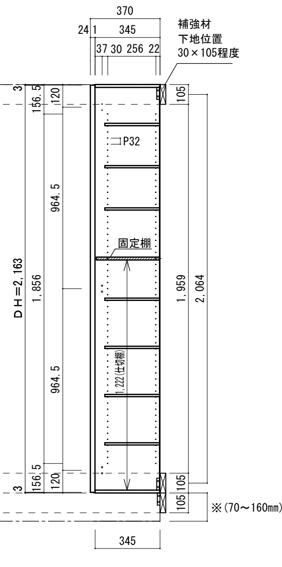
A-A' 断面図
