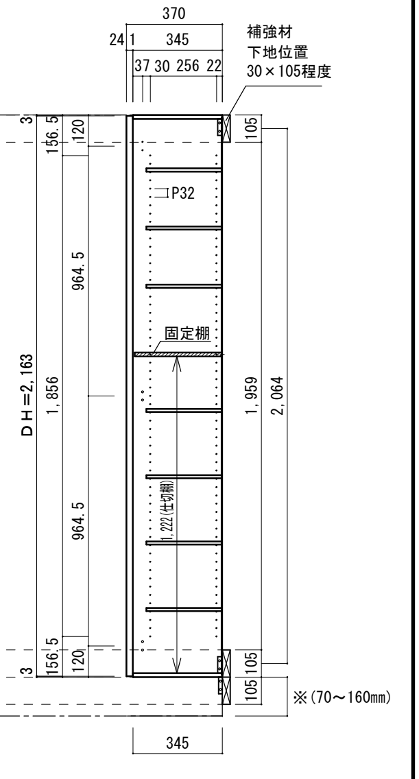
A-A' 断面図
