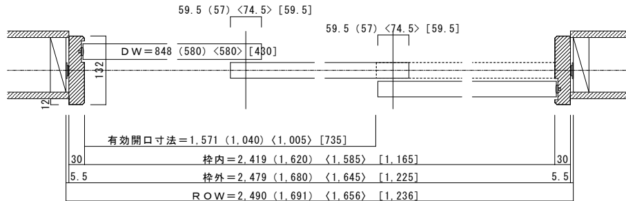
■横断面図 間口9尺 (6尺大) <6尺小> [4.5尺]
