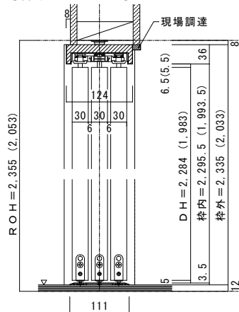
■縦断面図 H=8尺 (H=7尺)
