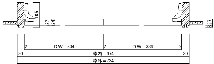
■横断面図 H=4尺、3尺
