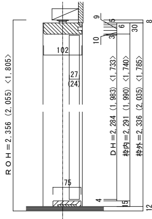
■縦断面図 H=8尺 (7尺) <6尺
