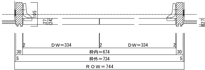
■横断面図 H=8尺、7尺、6尺
