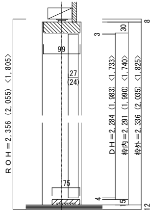
■縦断面図 H = 8尺 (7尺) < 6尺
