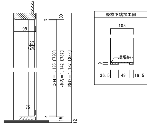
■縦断面図 H = 4尺 (3尺)
