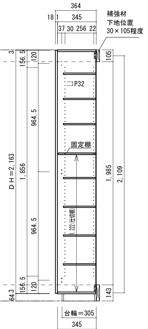
A-A' 断面図
