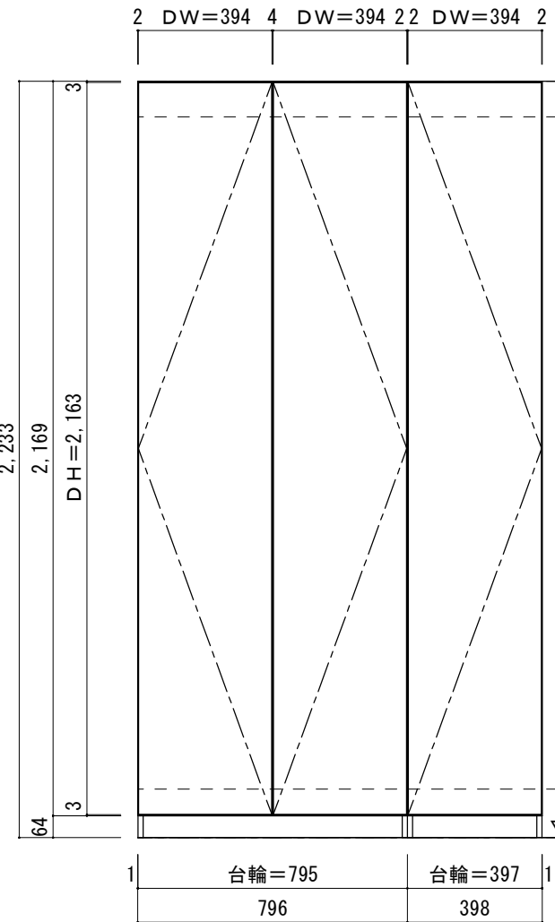
扉配置図
