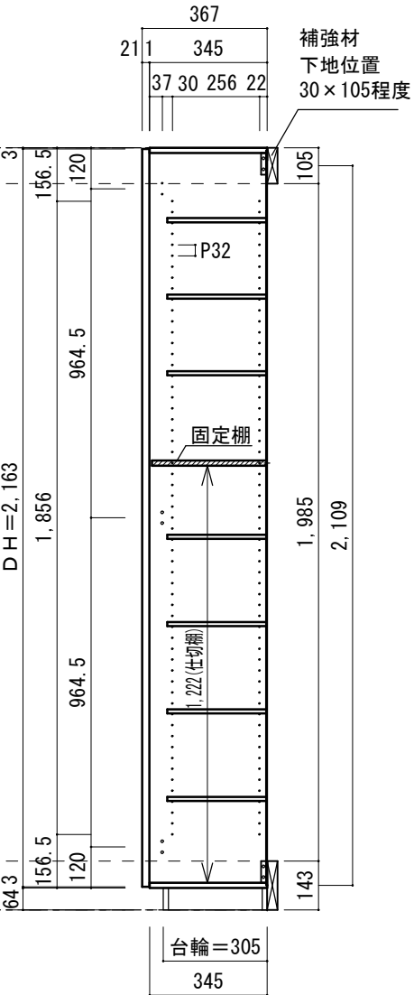
A-A' 断面図
