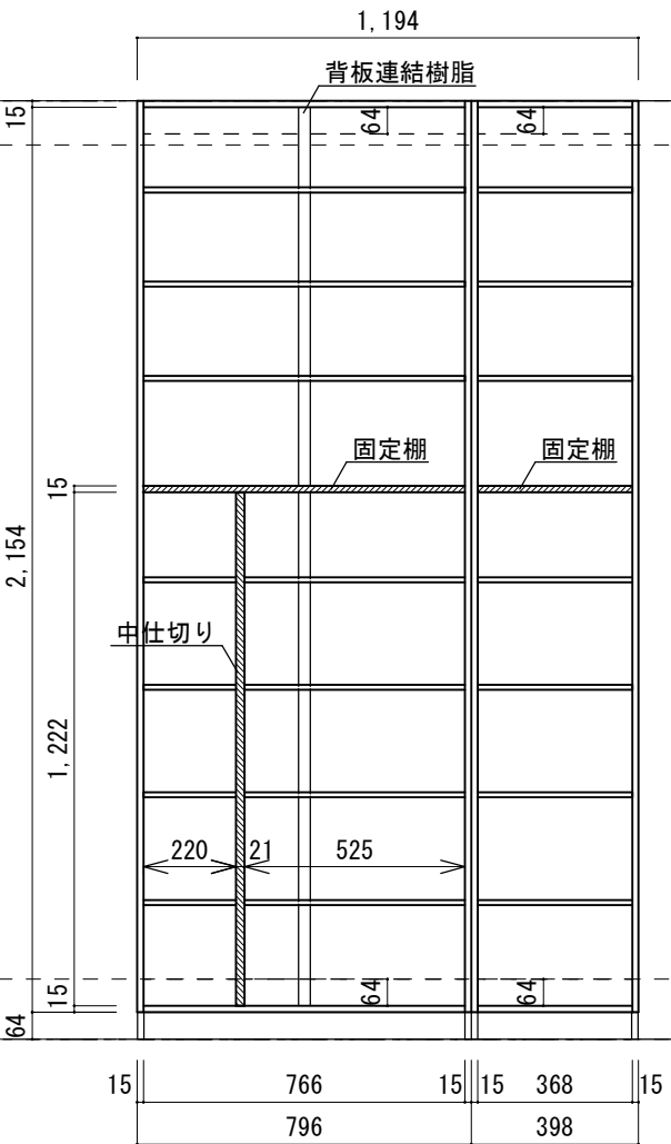
キャビネット図
