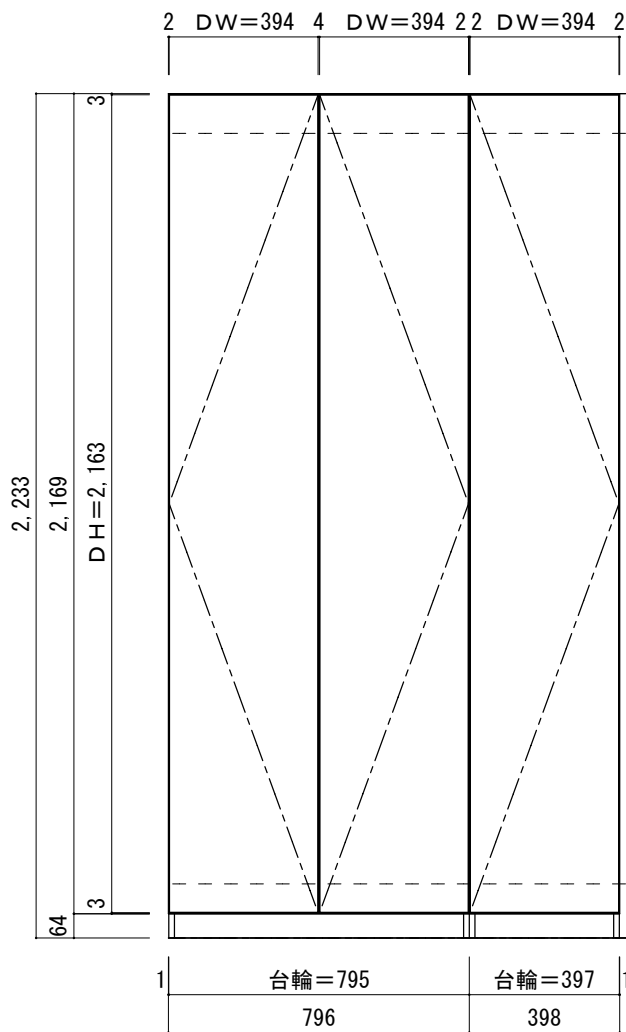
扉配置図
