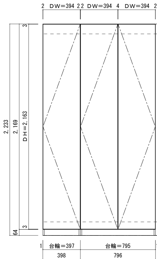
扉配置図
