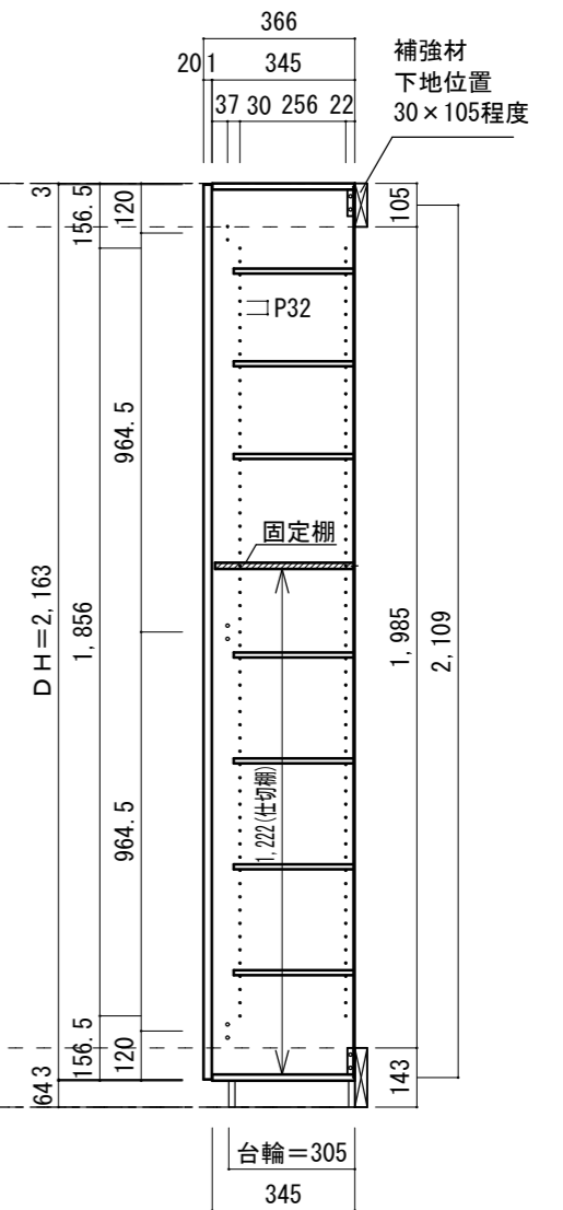
A-A' 断面図
