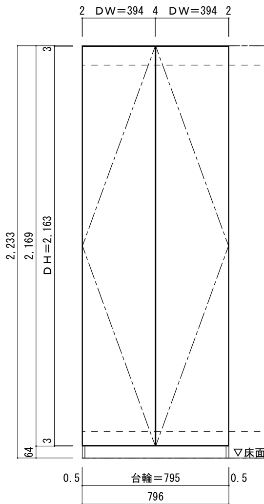
扉配置図
