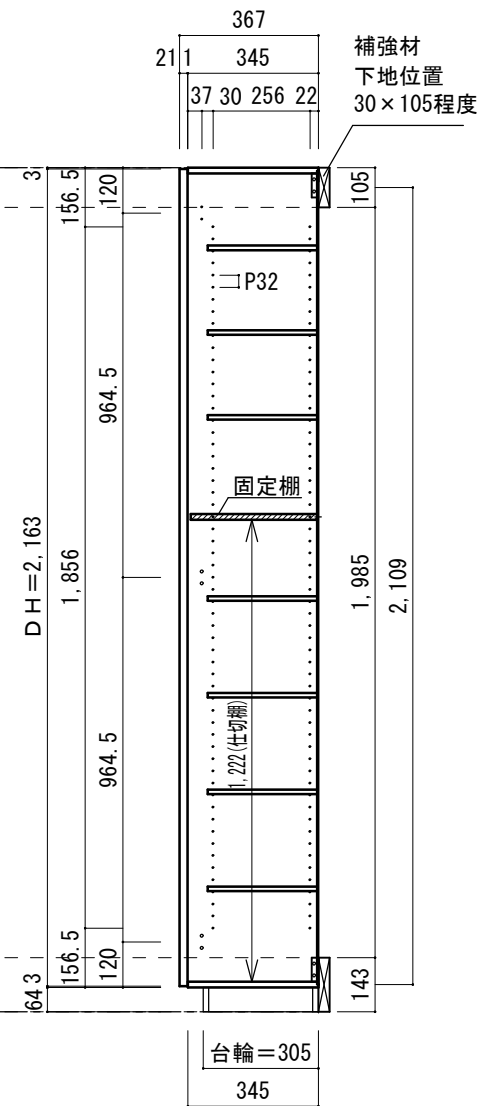
A-A' 断面図
