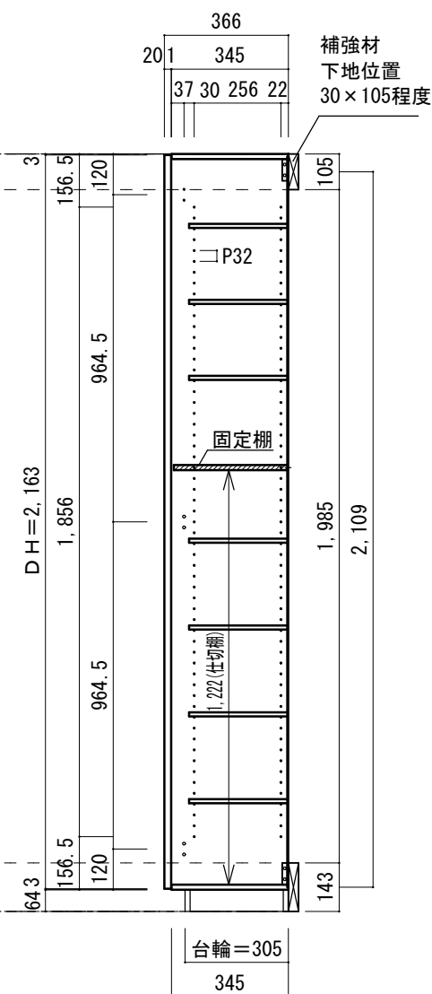
A-A' 断面図
