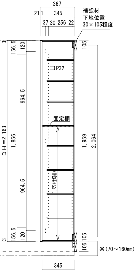
A-A' 断面図
