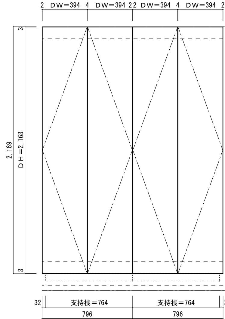
扉配置図
