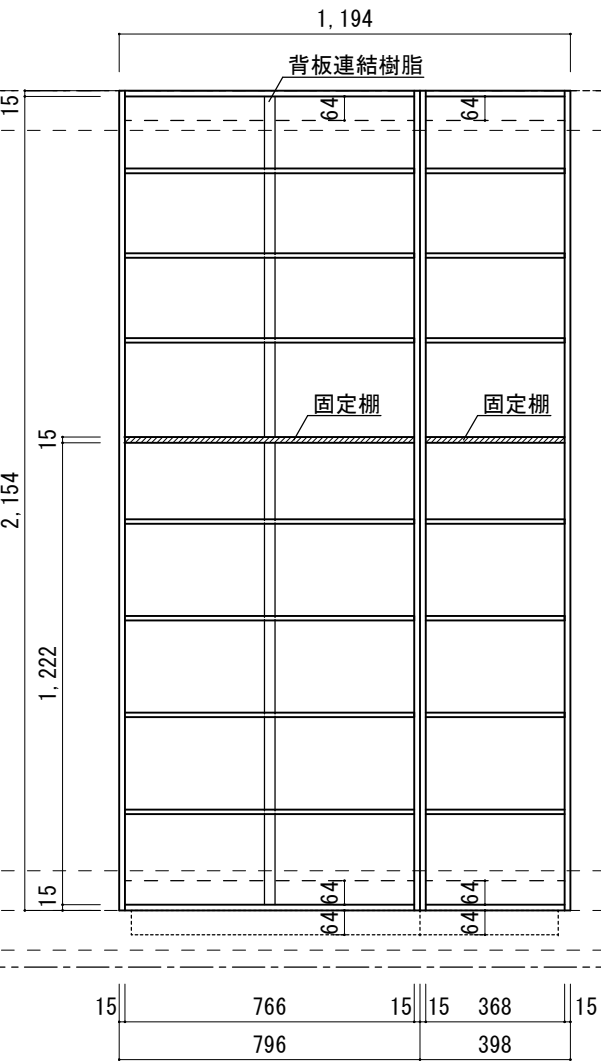
キャビネット図
