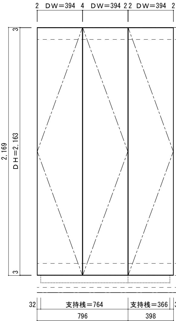
扉配置図
