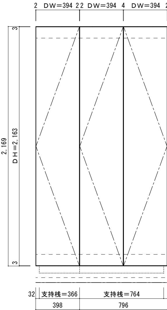
扉配置図
