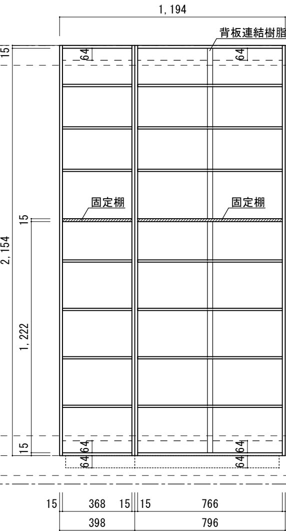
キャビネット図
