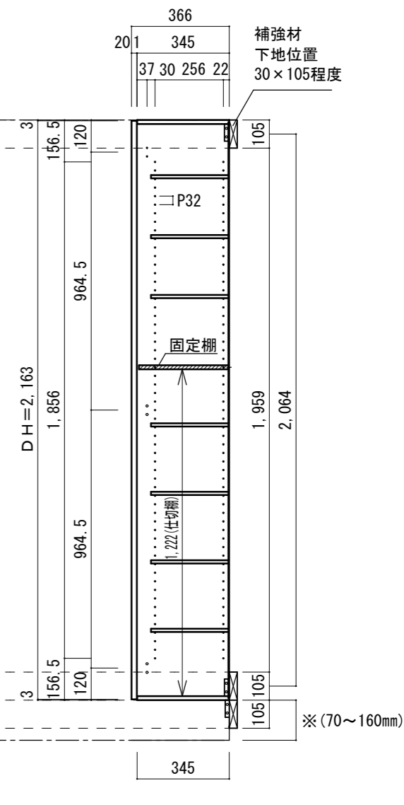
A-A' 断面図
