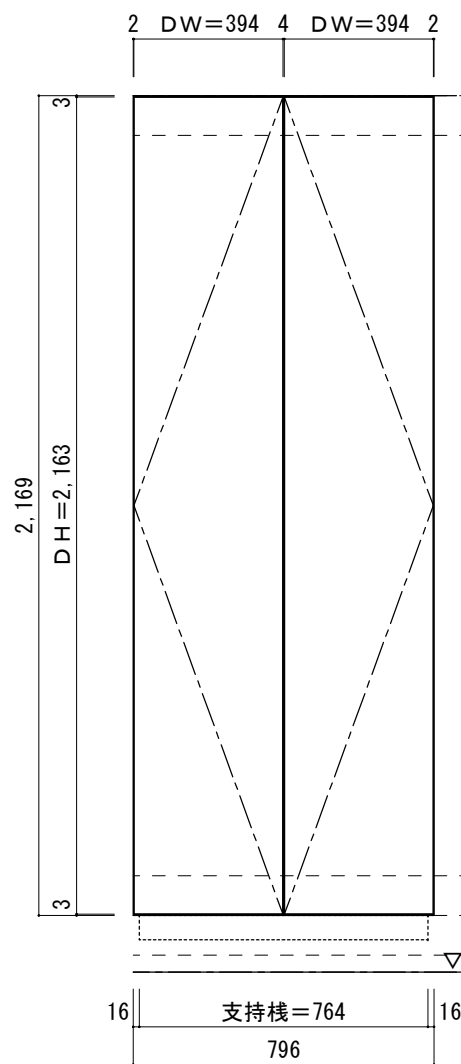
扉配置図
