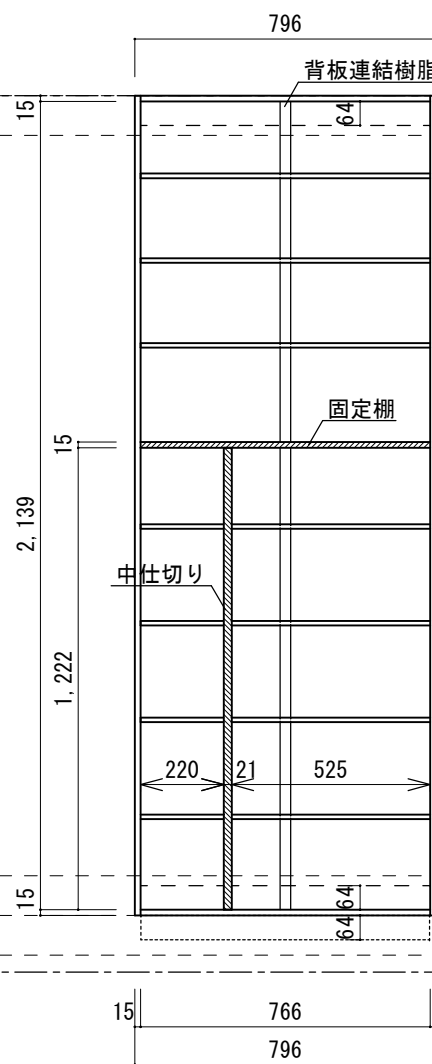
キャビネット図
