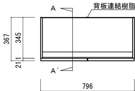
平面図
