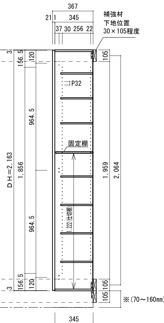
A-A' 断面図
