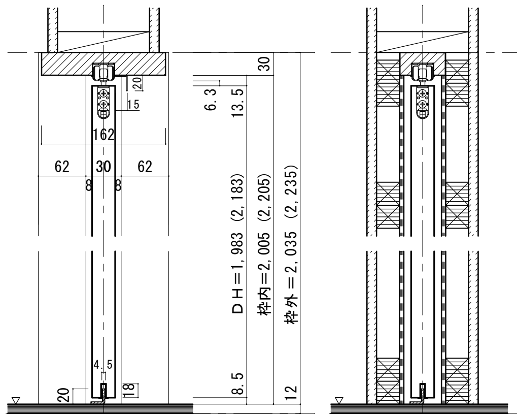
■縦断面図
