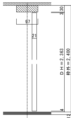
■縦断面図
