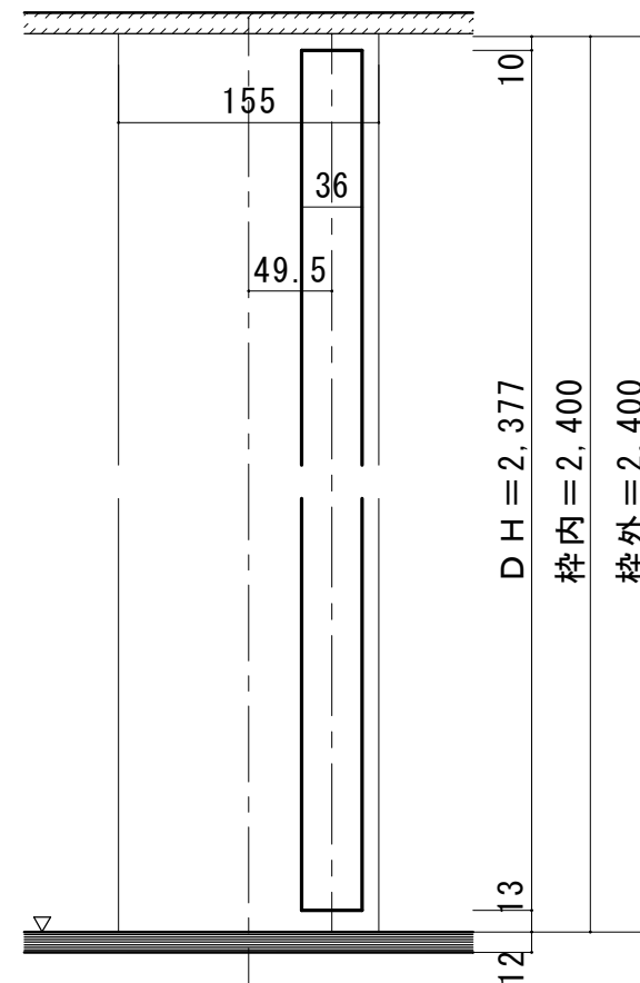
■縦断面図[2方枠]
