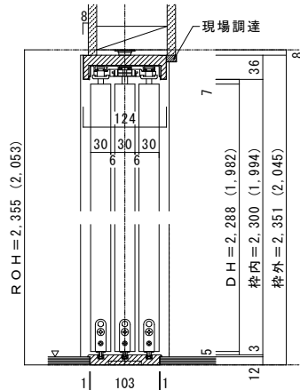
■縦断面図 H=8尺 (H=7尺) [レールタイプ]
