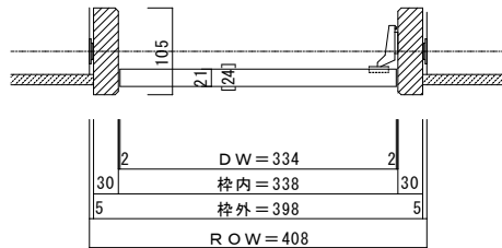
■横断面図 H=8尺、7尺、6尺
