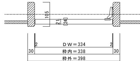
■横断面図 H=4尺、3尺
