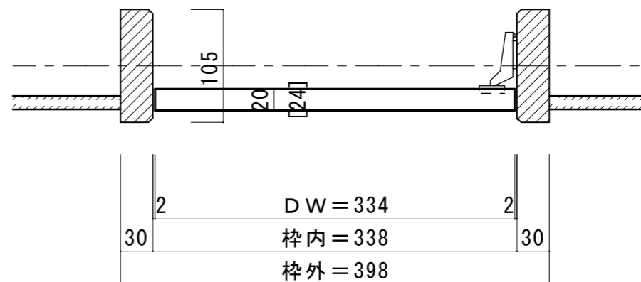
■横断面図 H=4尺、3尺
