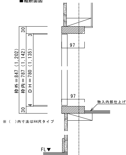
■縦断面図
