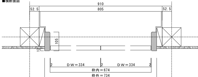
■横断面図
