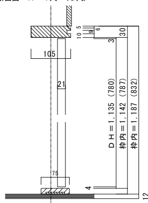
■縦断面図 H=4尺 (3尺)
