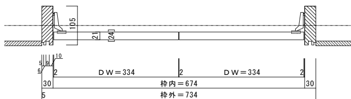
■横断面図 H=4尺、3尺
