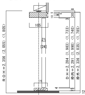
■縦断面図 H=8尺 (7尺) <6尺>
