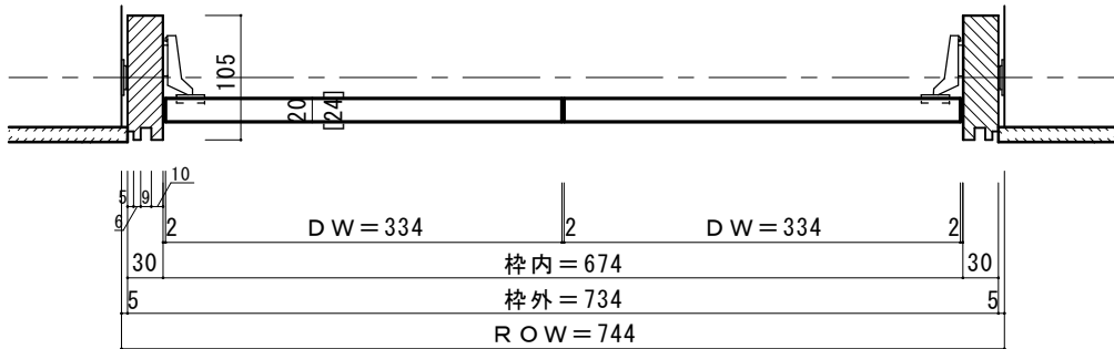
■横断面図 H=8尺、7尺、6尺
