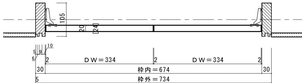
■横断面図 H=4尺、3尺
