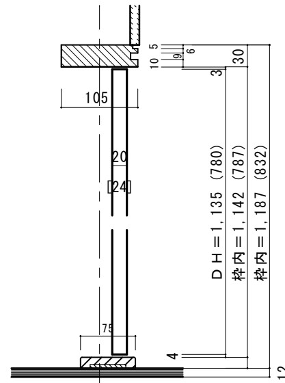
■縦断面図 H=4尺 (3尺)
