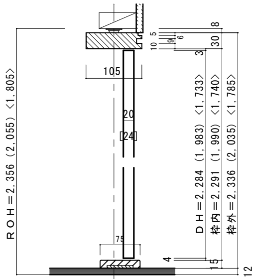
■縦断面図 H=8尺 (7尺) <6尺>
