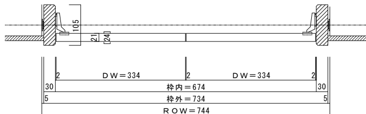
■横断面図 H=8尺、7尺、6尺
