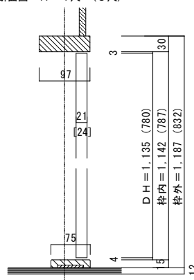
■縦断面図 H=4尺 (3尺)
