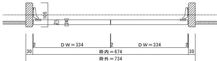
■横断面図 H=4尺、3尺
