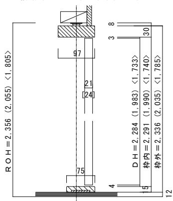
■縦断面図 H=8尺 (7尺) <6尺>
